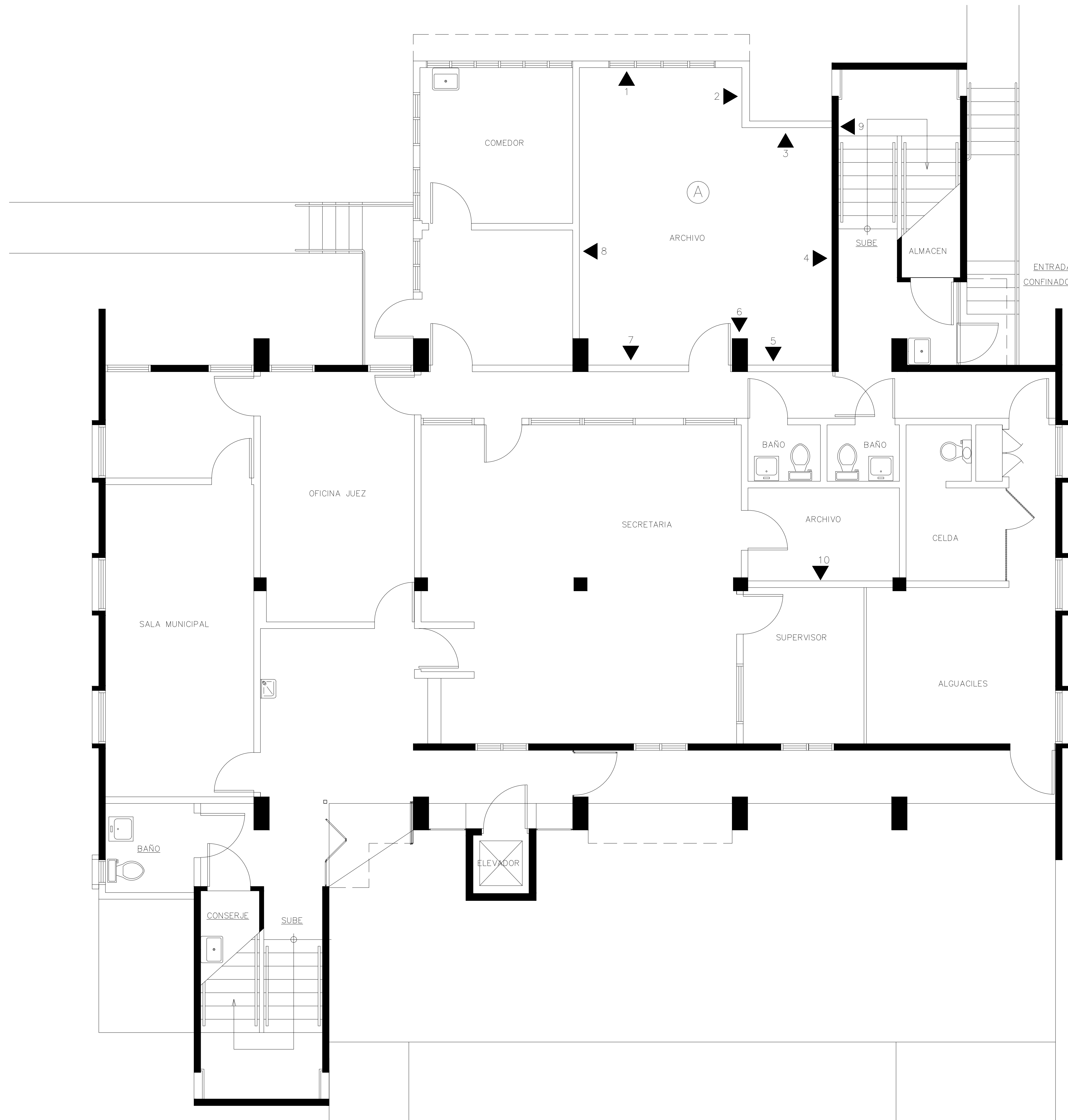
PLANO RESTAURACIÓN Y MEJORAS TPI AÑASCO PISO 1 ESCALA: 1/4"=1'-0"
