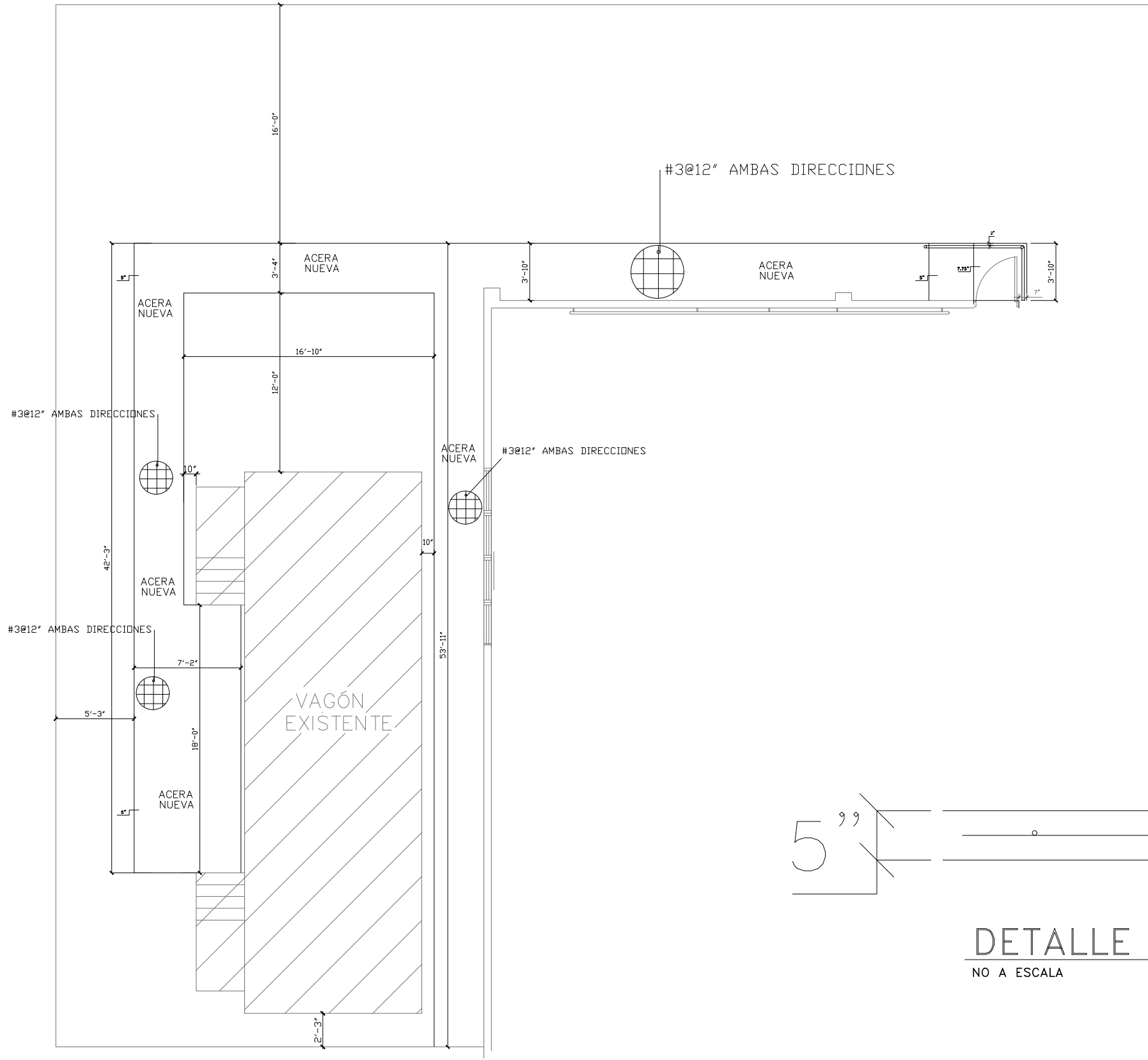
PLANO ESTRUCTURAL ESCALA: 1/4" = 1'-0"
