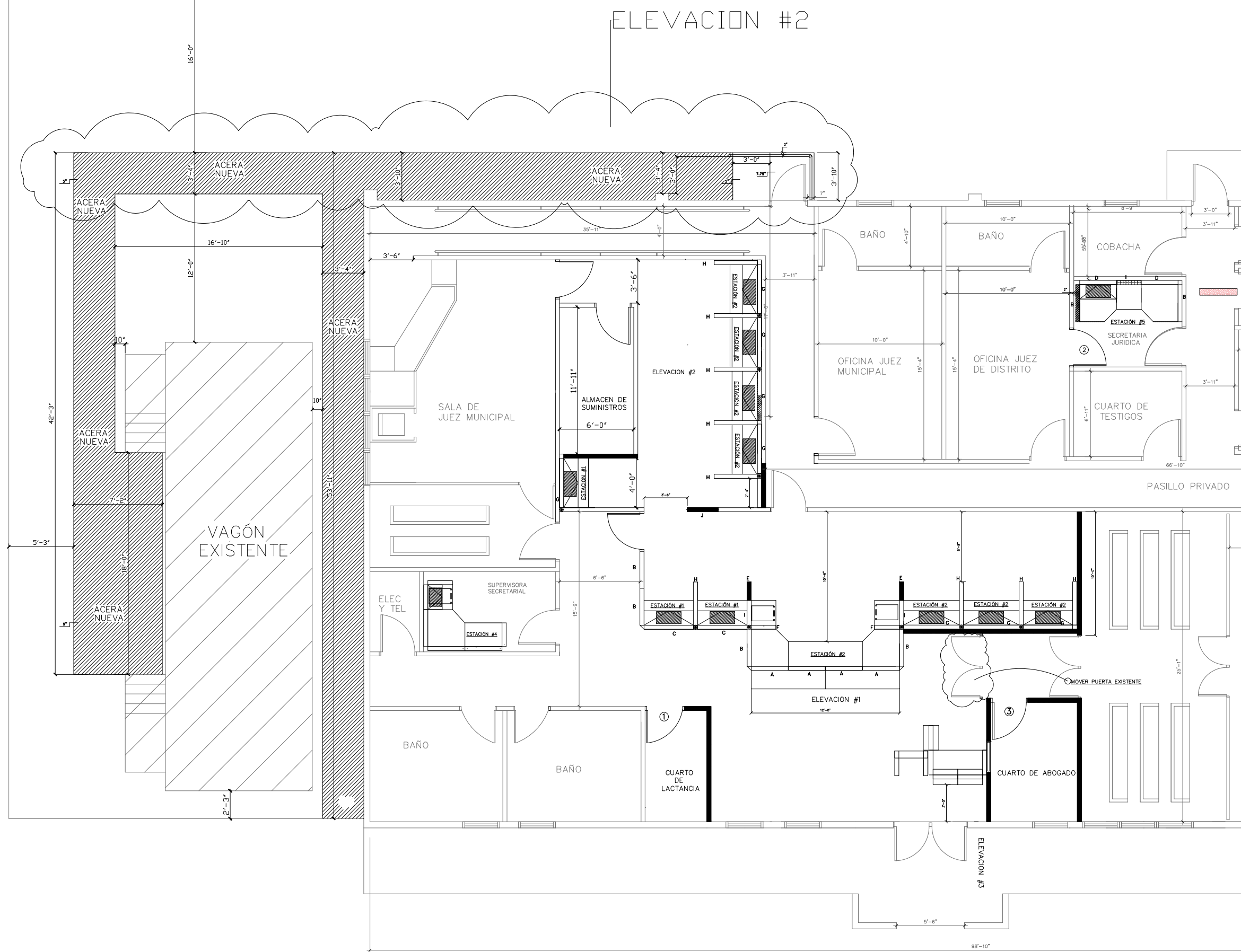
PLANO DE CONSTRUCCION NUEVO ESCALA: 1/4" = 1'-0"
