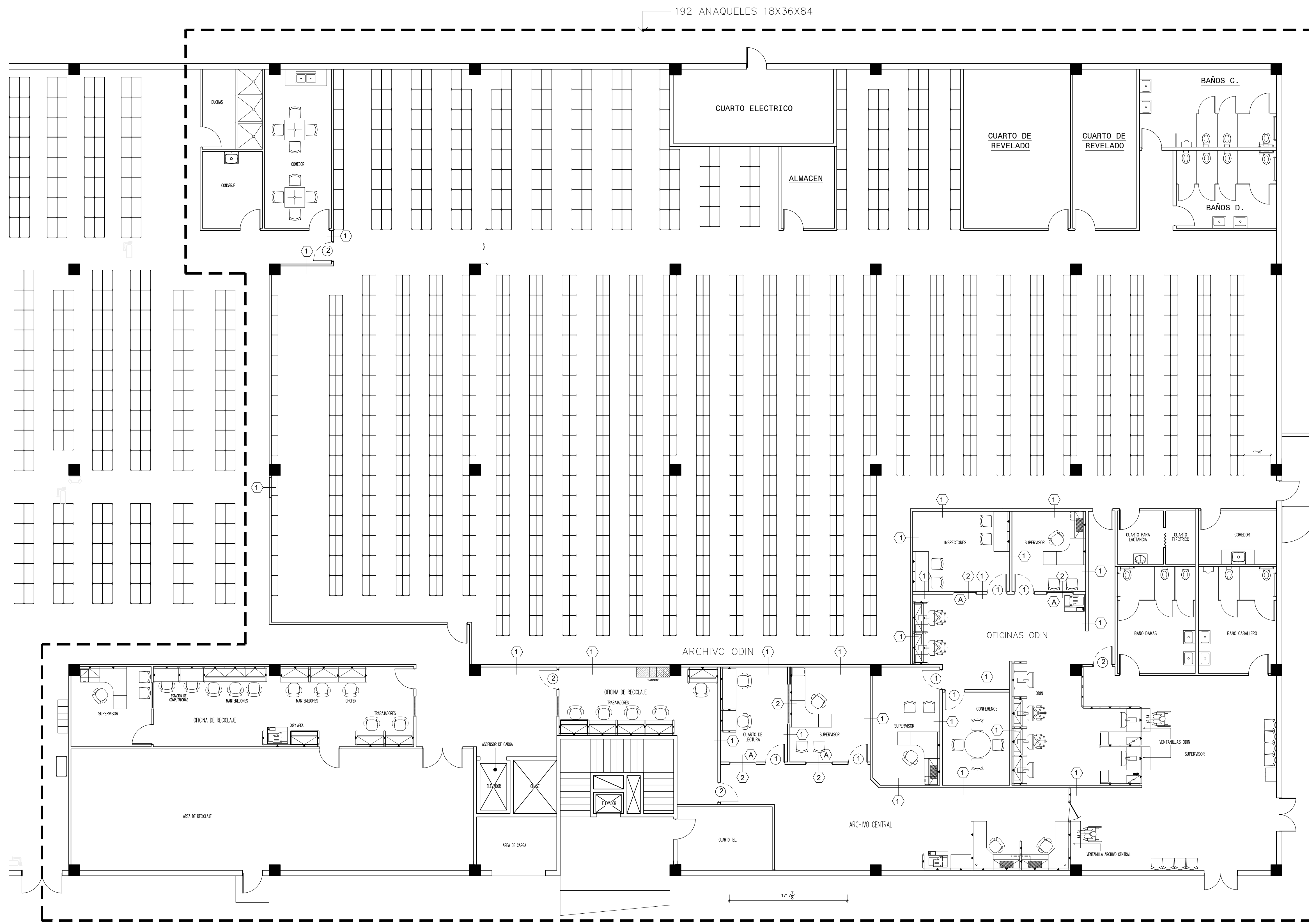
PLANTA PROPUESTA scale: 1/8" = 1'-0"
