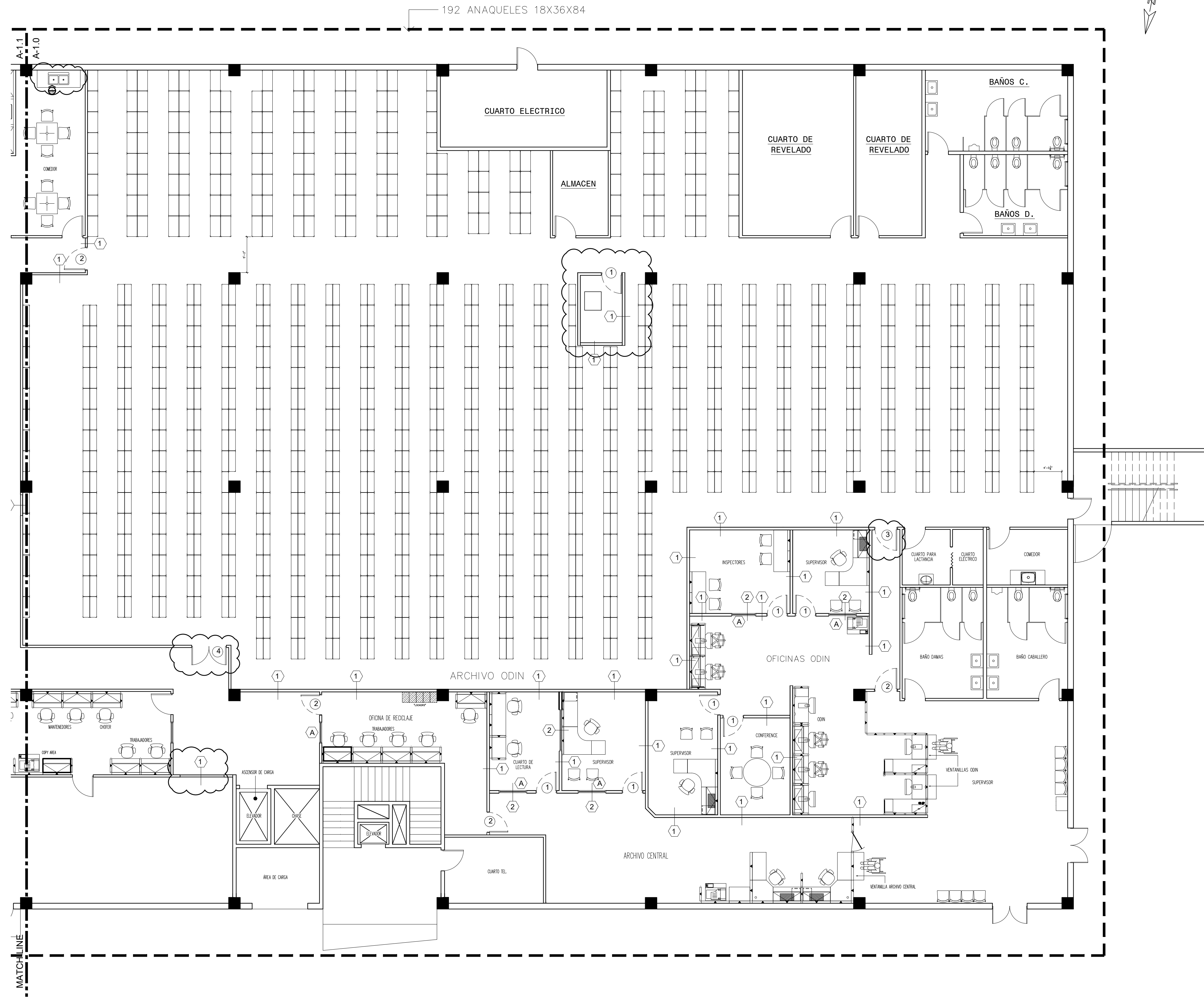
PLANTA PROPUESTA scale: 1/8" = 1'-0"
