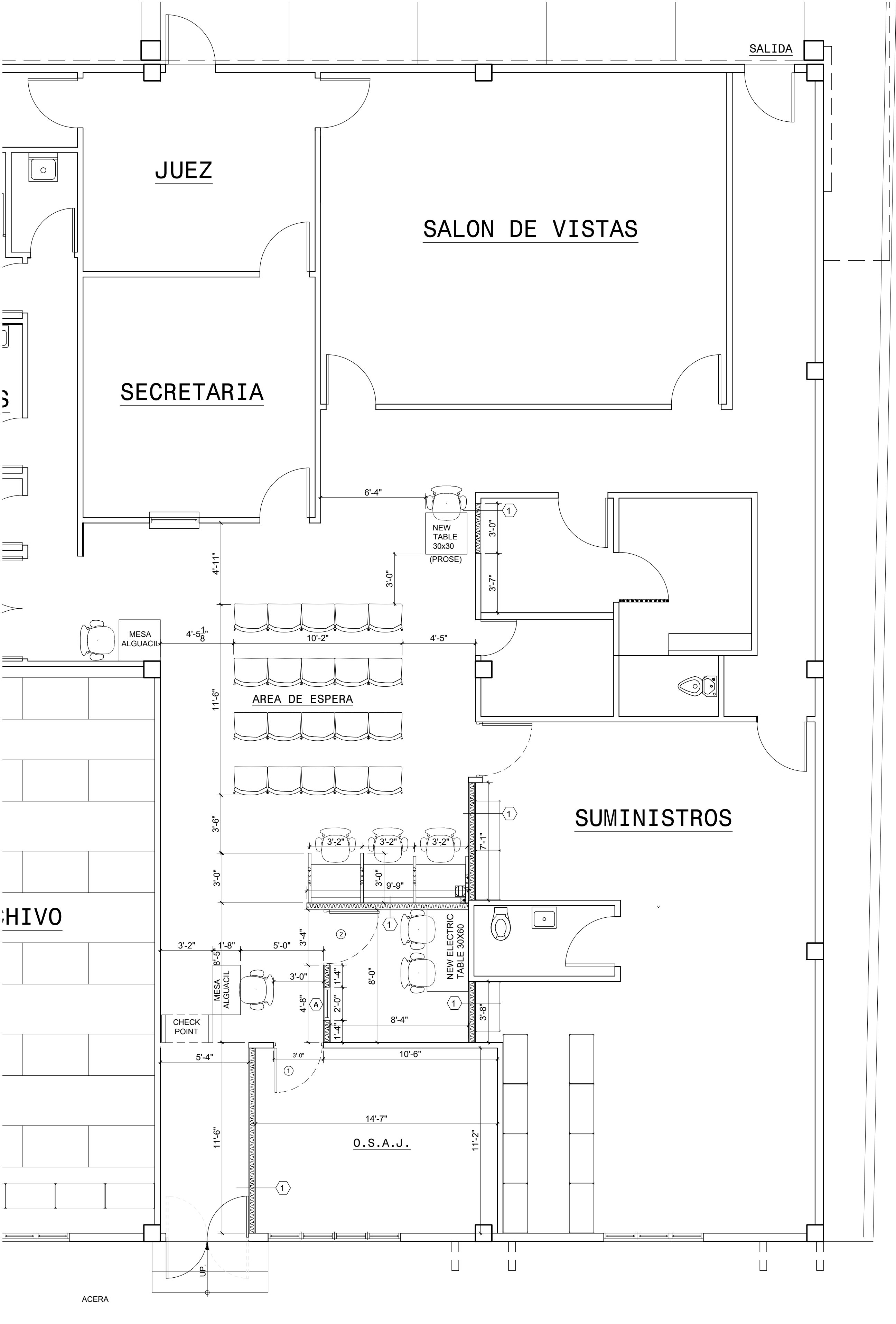
PLANTA PROPUESTA SUMAC MUNICIPAL CJ-AIBONITO SCALE: 1/4"=1'-0"
