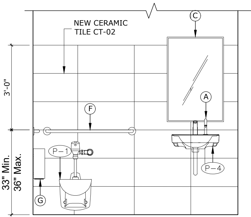
ELEVATION 2 SCALE: 3/8"=1'-0"
