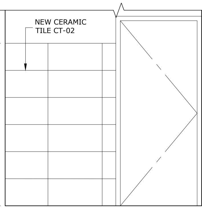
ELEVATION 3 SCALE: 3/8"=1'-0"
