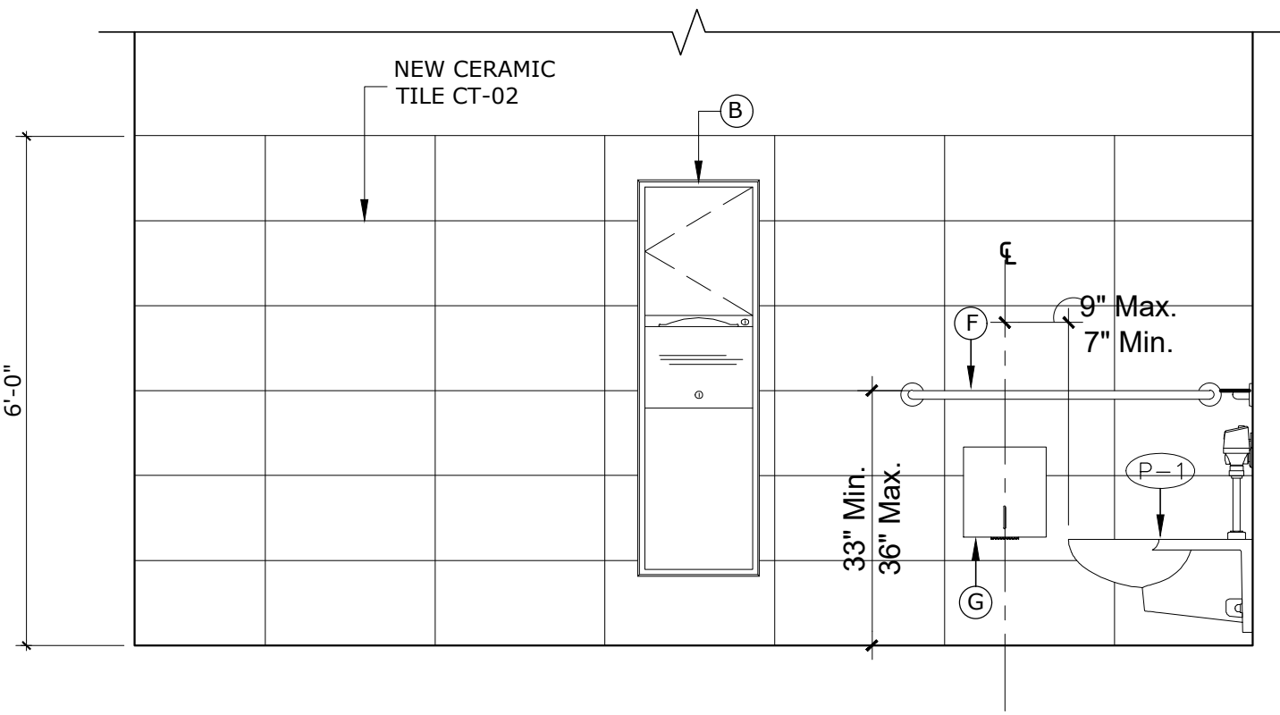
ELEVATION 1 SCALE: 3/8"=1'-0"
