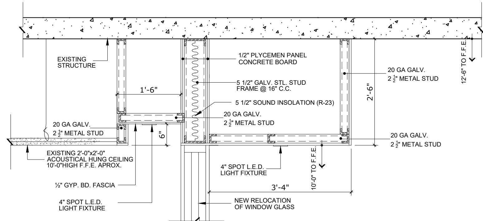
DETAIL SCALE: 3/4"=1'-0"
