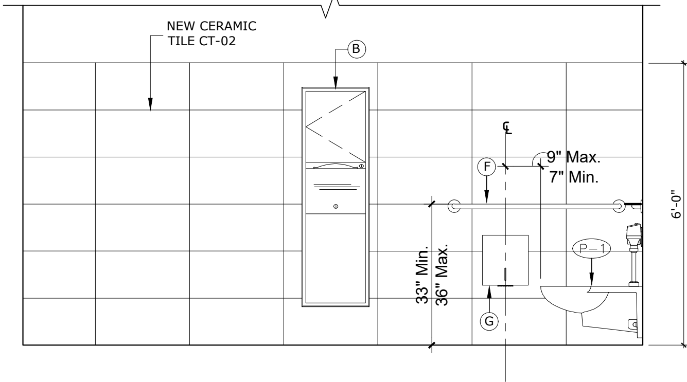
ELEVATION 1 SCALE: 3/8"=1'-0"
