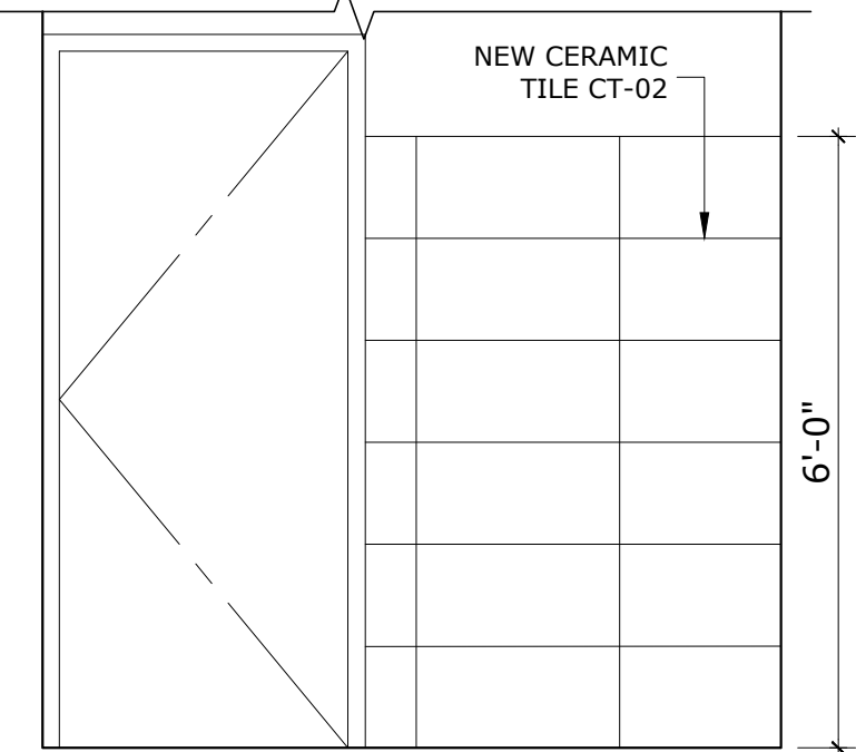
ELEVATION 3 SCALE: 3/8"=1'-0"
