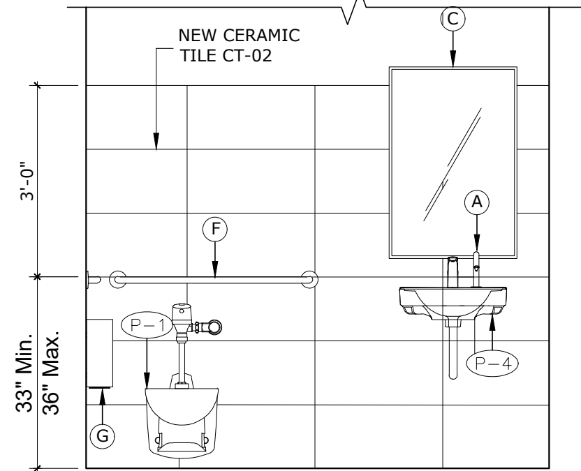
ELEVATION 2 SCALE: 3/8"=1'-0"
