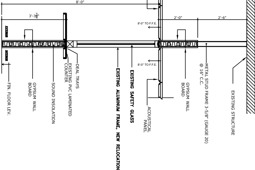
DETAILE DE PARED TIPO 2
