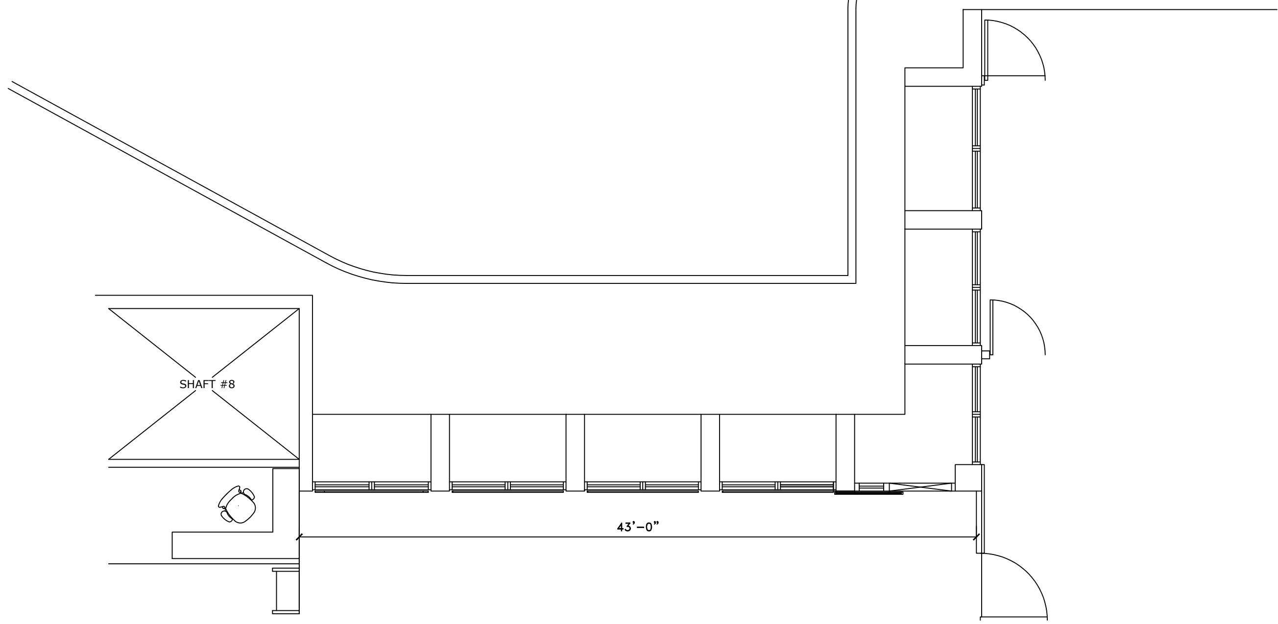
CJSJ - SOTANO - AREA DE SALA DE INVESTIGACIONES ESCALA: 3/8" = 1'-0"
