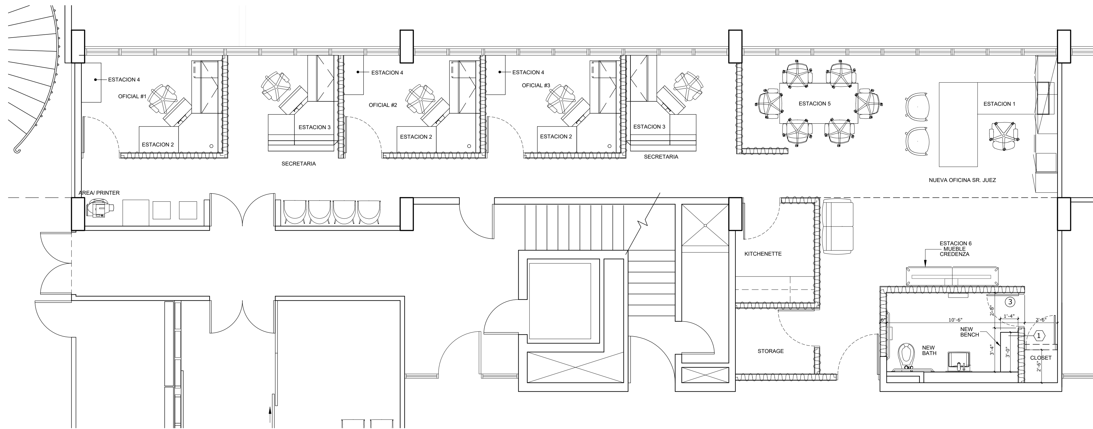
MOBILIARIO NUEVA OFICINA, SCALE: 3/16"=1'-0"
