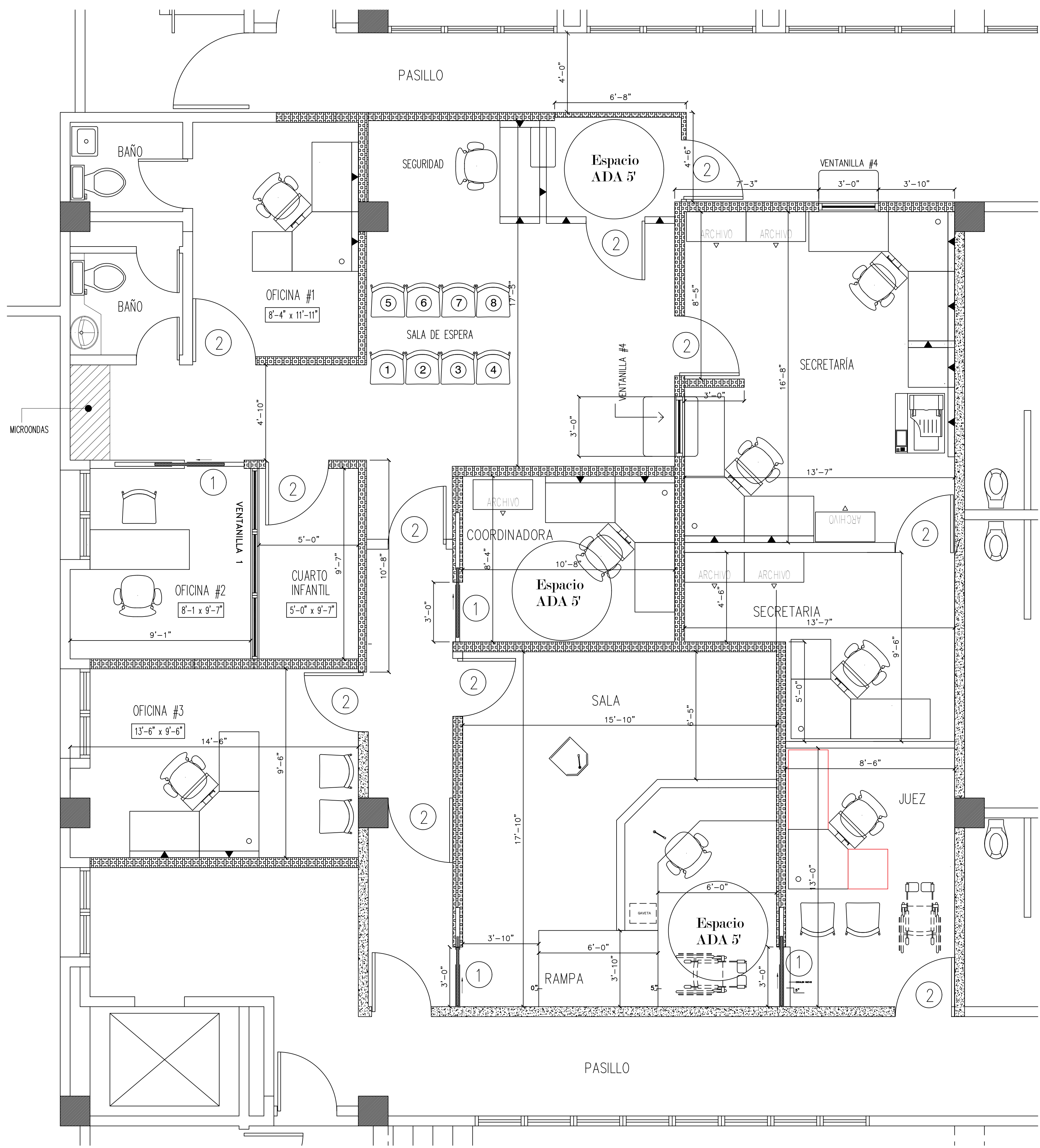
PLANTA DE PISO PROPUESTO ESCALA: 3/8" = 1'-0"
