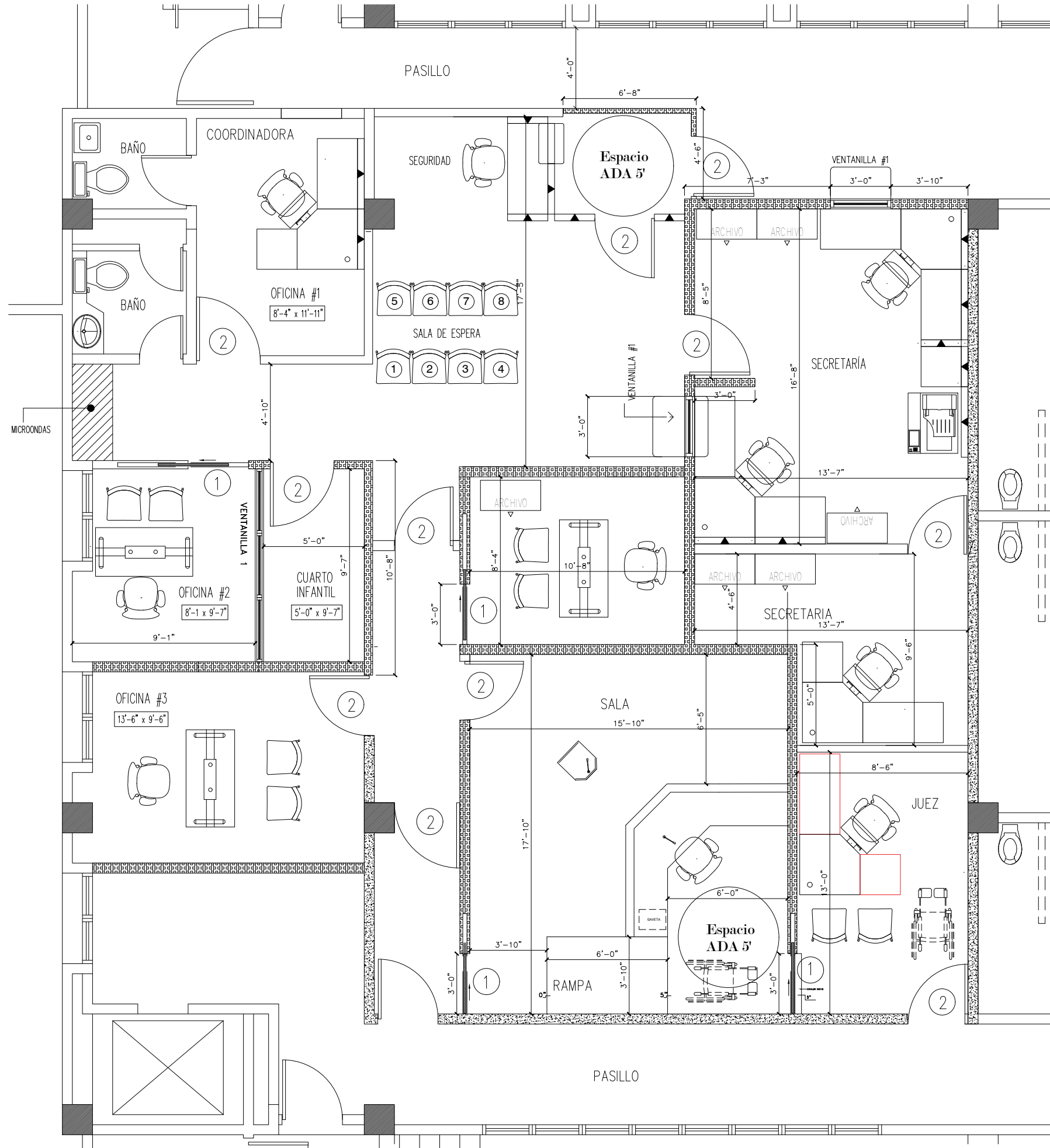
PLANTA DE PISO PROPUESTO ESCALA: 3/8" = 1'-0"
