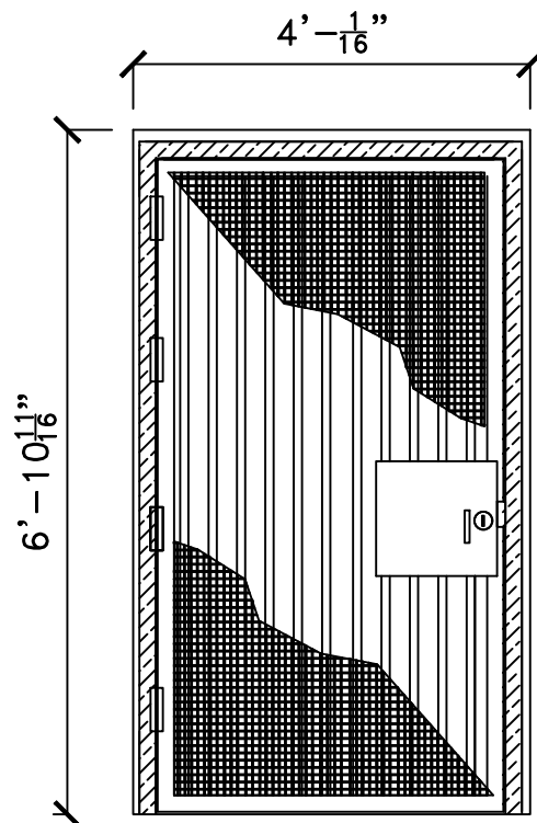
PISO 5 LADO IZQUIERDO PORTÓN CON MARCO VISTA EXTERIOR LLAVE DE AMBOS LADOS ESCALA: 1" = 1'-0" MARCO
