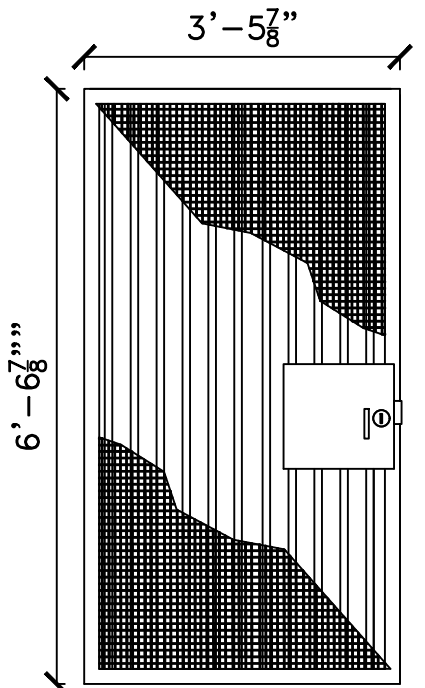
PISO 5 LADO IZQUIERDO LLAVE DE AMBOS LADOS PORTÓN SOLO ESCALA: 1" = 1'-0"
