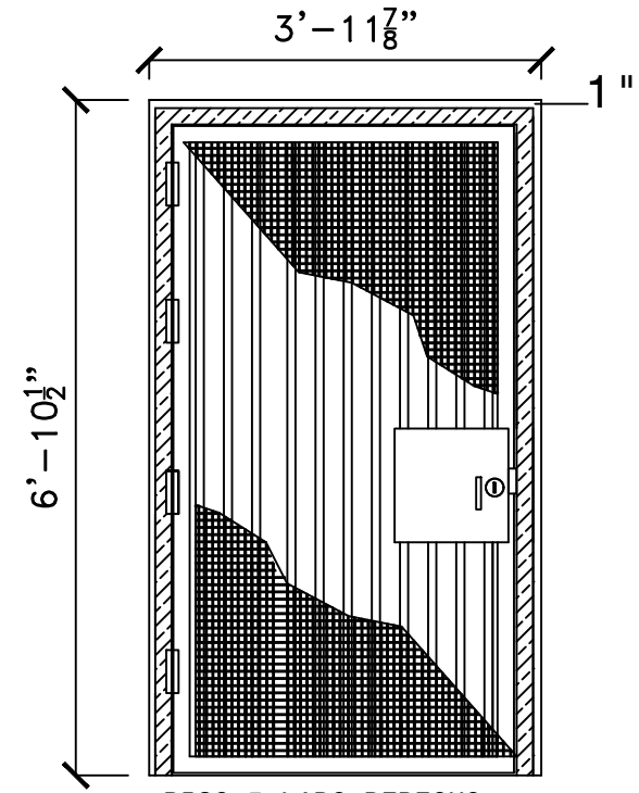
PISO 5 LADO DERECHO PORTÓN CON MARCO LLAVE DE AMBOS LADOS VISTA EXTERIOR ESCALA: 1" = 1'-0" MARCO
