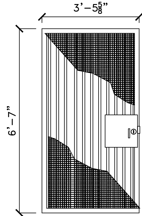
PISO 5 LADO DERECHO PORTÓN SOLO LLAVE DE AMBOS LADOS ESCALA: 1" = 1'-0"
